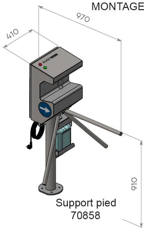
Version droite 70856
