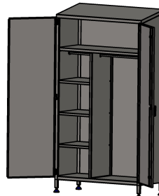
ARMOIRE AK 3 + Cloison + Etagere 1/3 Code : 3899 Code : 8155 Code : 8159
